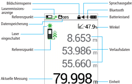
PIC1 Hauptoberfläche
